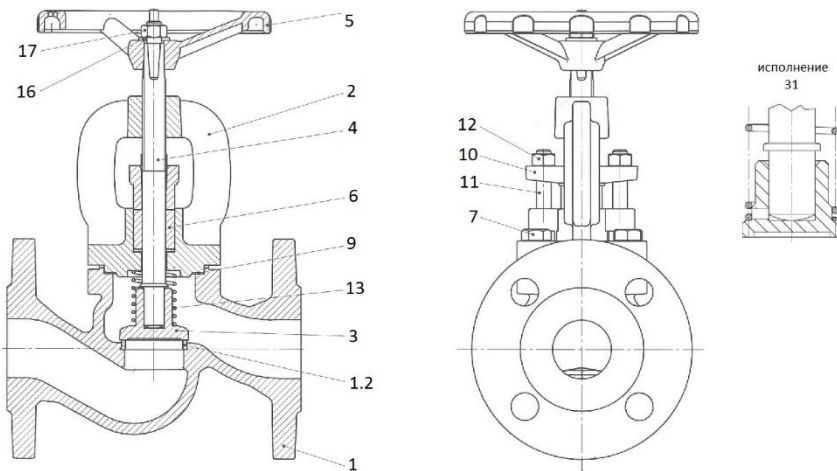
Клапан 215 [A] запорно-обратный
